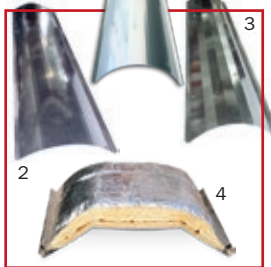
Parabola 1 standard - 2 ad alto rendimento - 3 a 7 facce - 4 a 3 facce con lana di vetro (in basso) Reflector 1 standard - 2 Highly efficient - 3 7-face - 4 3-face with glass wool (bottom)
